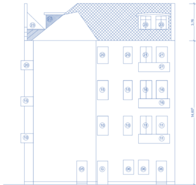
Ostansicht Dreiserstraße
